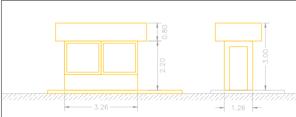
PROSPETTI CHIOSCO GESTORE (ESISTENTE) DA DEMOLIRE SCALA 1:100
