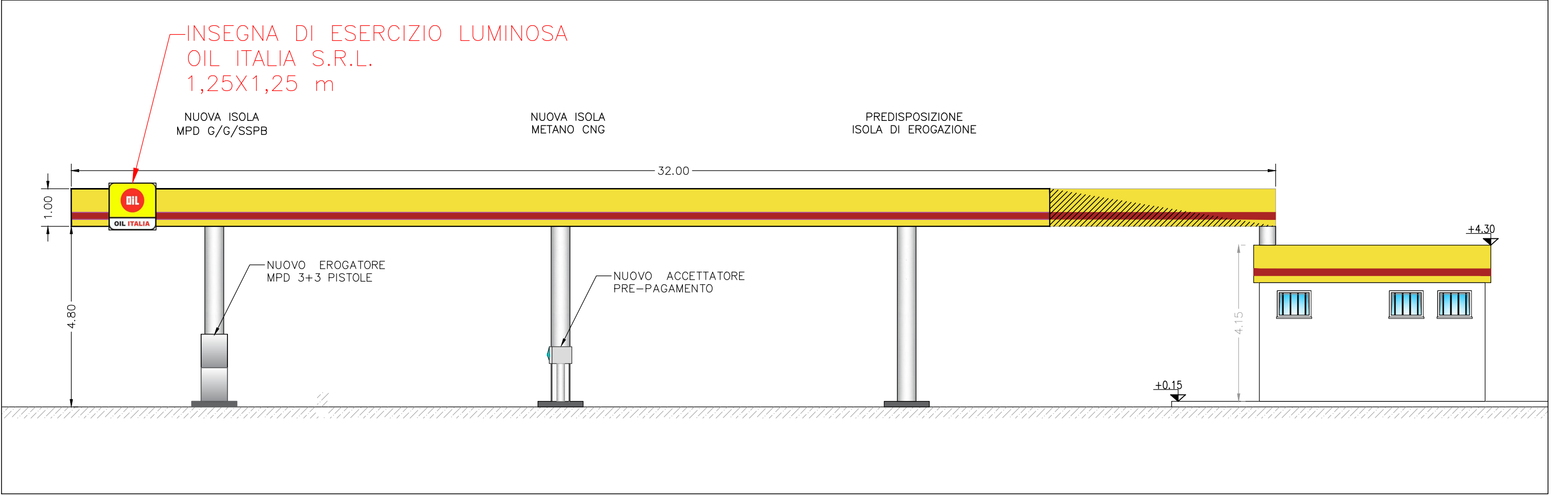
NUOVA PENSILINA – INDICAZIONE INSEGNA DI ESERCIZIO – SCALA 1:100
