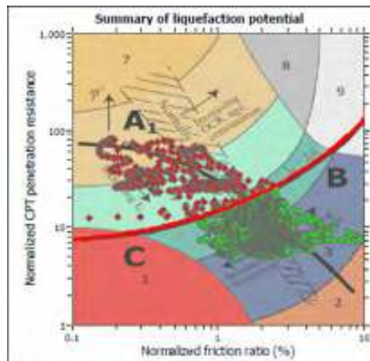
Plottaggio parametri CPTU 4 sulla Carta della classificazione di P.K. Robertson (1990; 2009).
