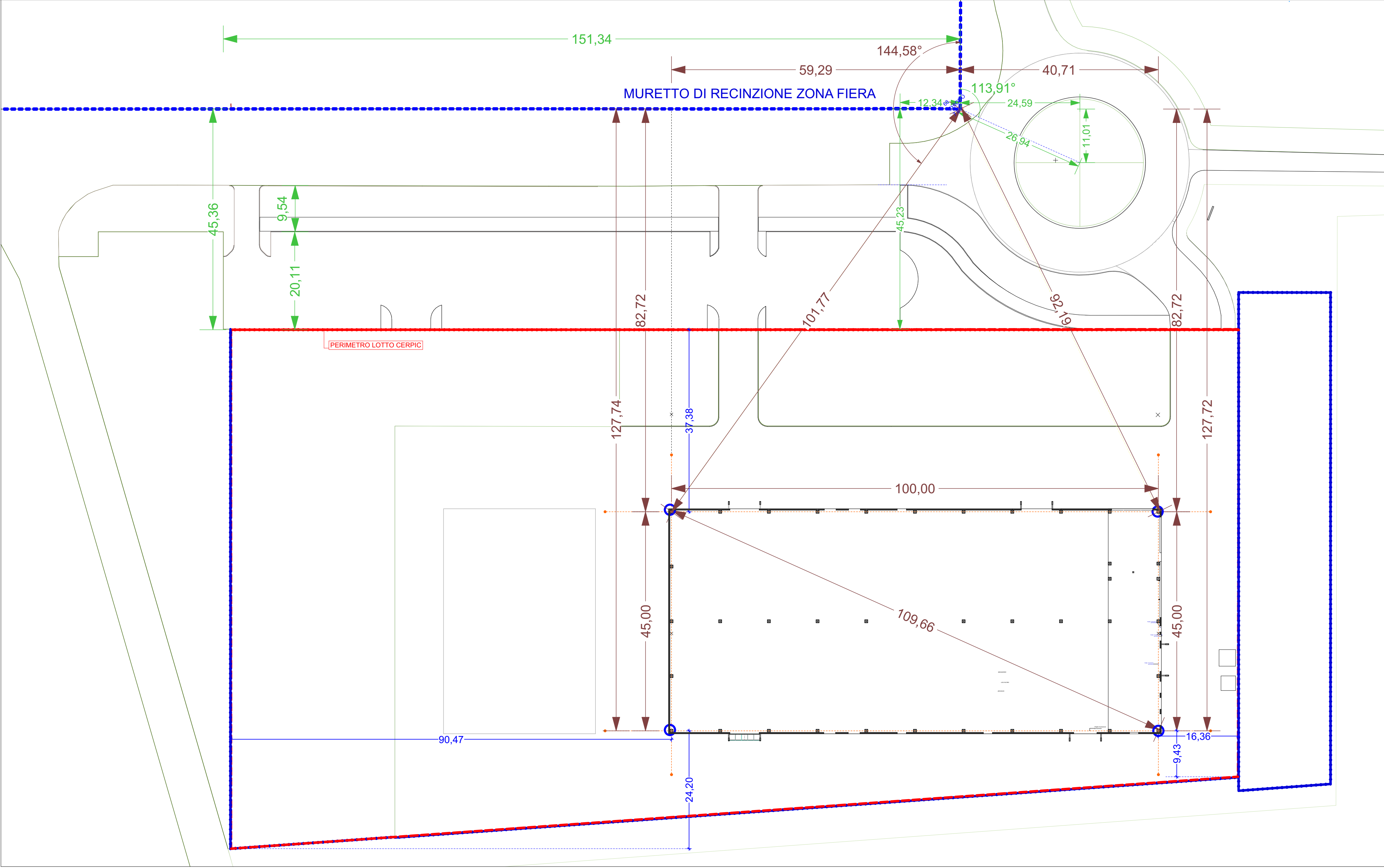
Tracciamento Fabbricato
