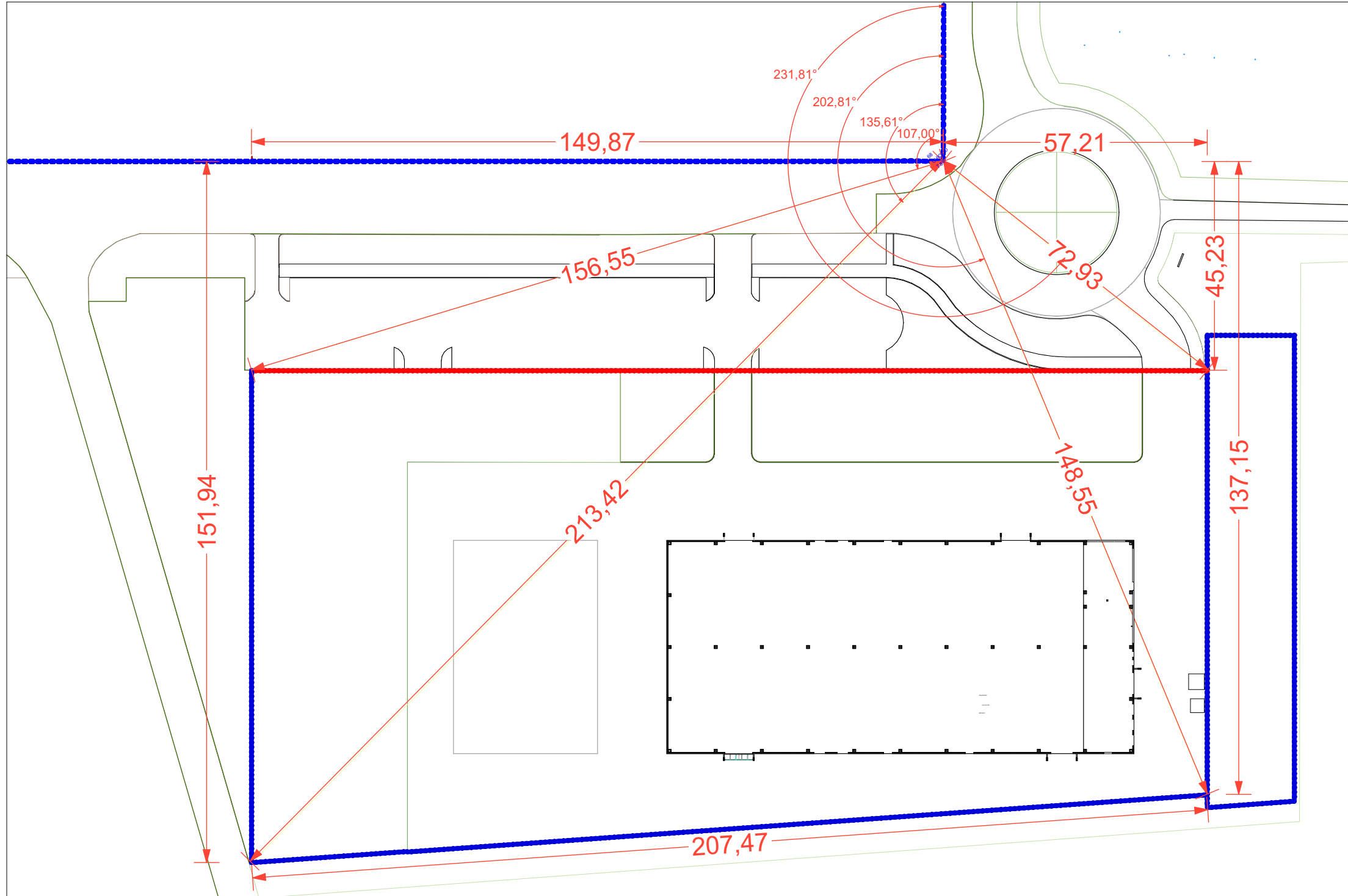
Tracciamento Lotto
