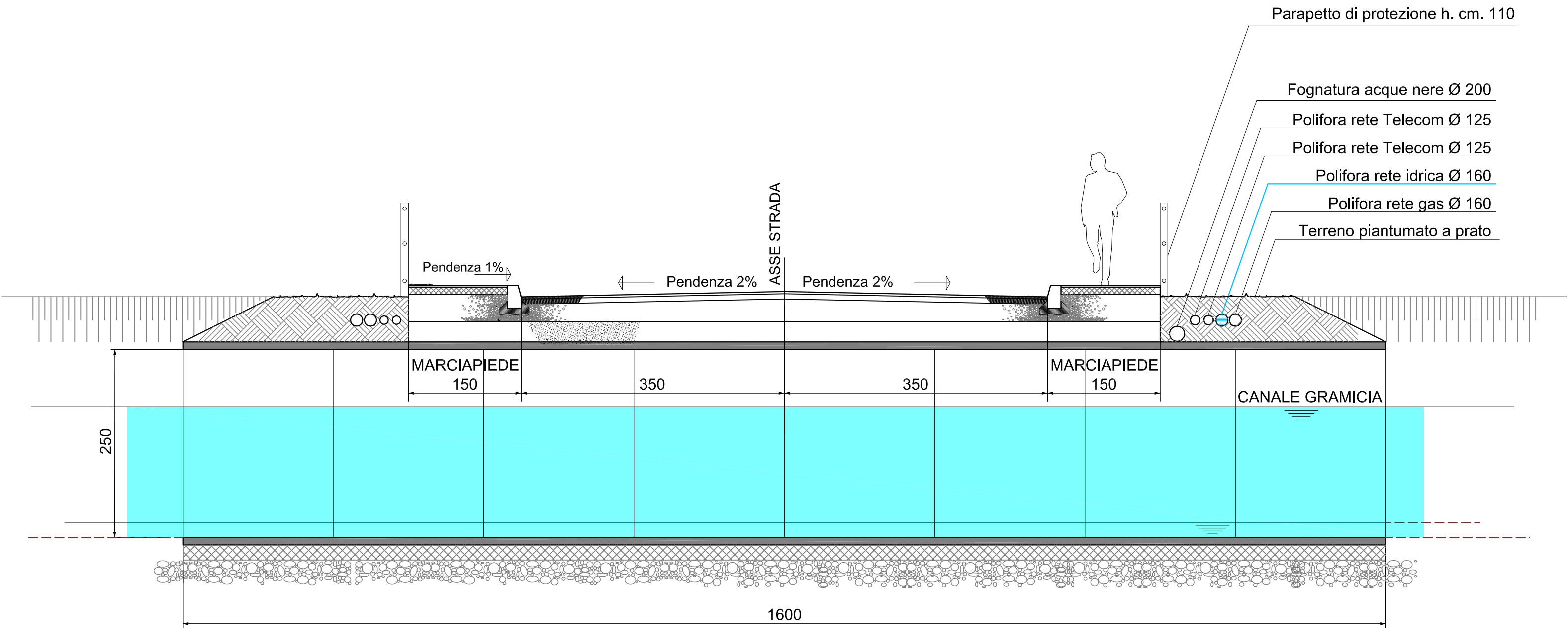
SEZIONE SUL PONTE DI PROGETTO Scala 1:50
