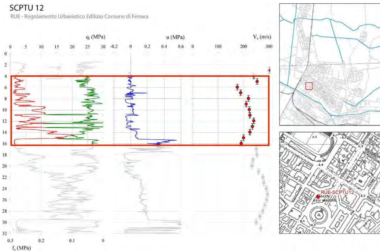
Figura 5-4 - Log parametrici di resistenza alla punta ( q_t ), attrito laterale ( f_s ), pressione neutra ( u ) e velocità delle onde sismiche secondarie ( V_s ) relativi al piezocono sismico realizzato in Piazza XIV Maggio, nell'ambito dei lavori per il R.U.E. -Regolamento Urbanistico Edilizio. L'andamento della resistenza alla punta ben riflette la sequenza positiva (finning up) delle sabbie e sabbie limose di riempimento del canale principale del Po di età antica e medioevale. Parte sommitale della successione corrisponde ad un riporto antropico.
