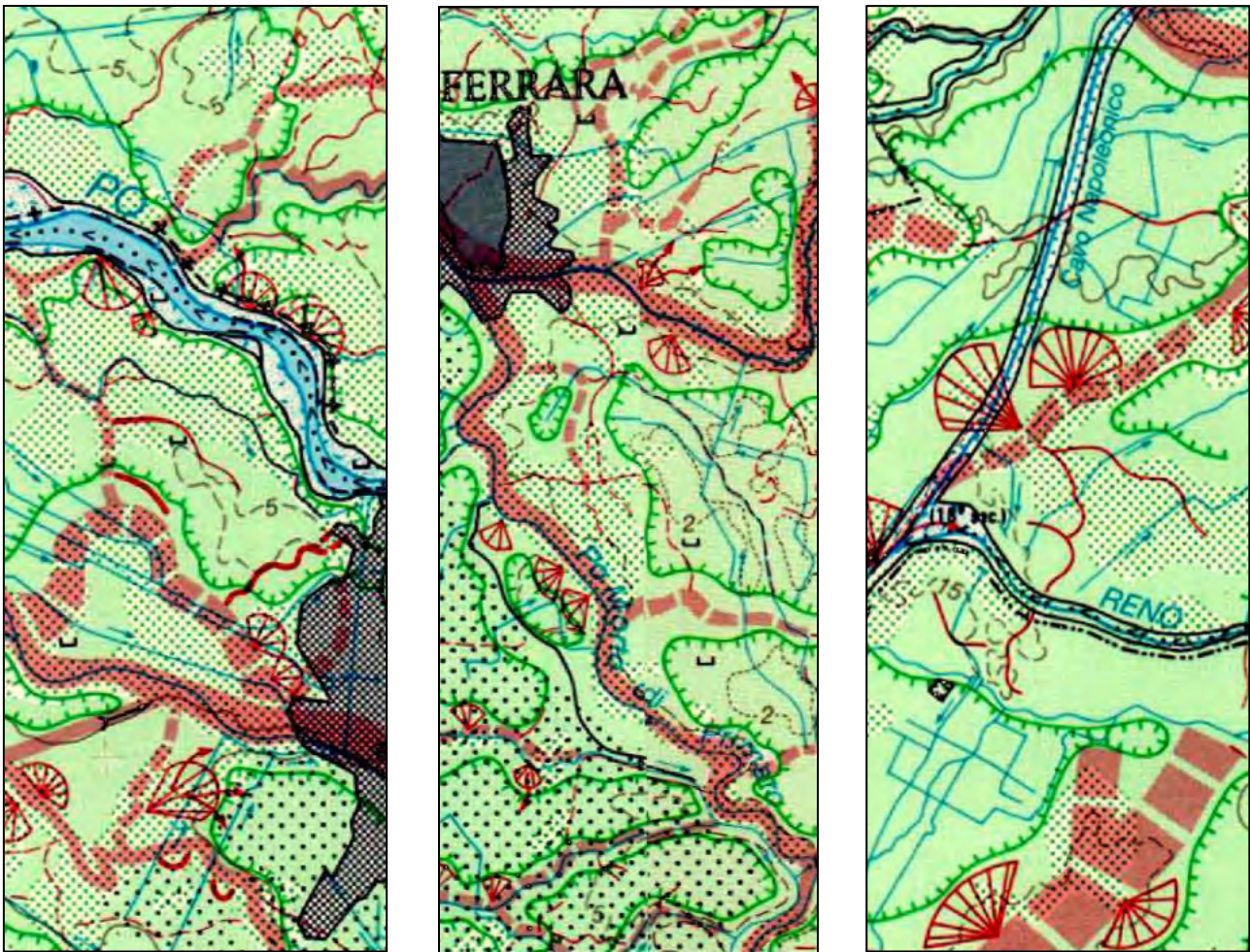
Figura 2-3 - Stralci della Carta Geomorfologica della Pianura Padana alla scala 1:250.000, rappresentanti aree ad ovest, sud-est e sud della città, in cui sono ben visibili dossi di paleoalveo di Po e di Reno.
