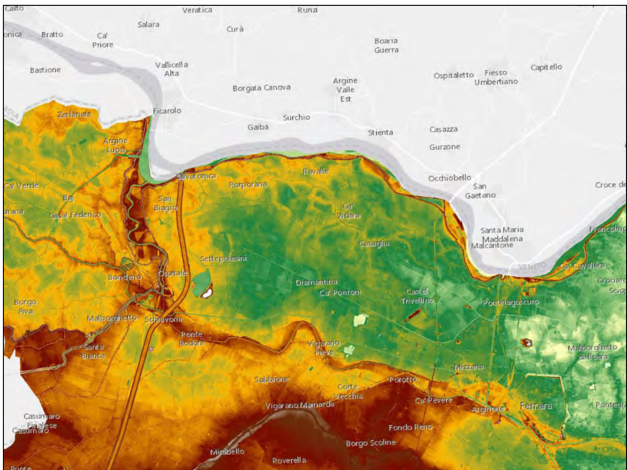
Figura 2-15 - Pianura a meandri a nord-ovest della città di Ferrara. I corpi di alveo meandriciforme non generano dossi pensili e presentano quindi una ridotta espressione morfologica. Forme planimetriche curvilinee, legate a meandri preistorici del Po, sono ben visibili fra Casaglia e Vigarano Pieve e nei pressi di Salvatonica, subito ad occidente del confine comunale.
