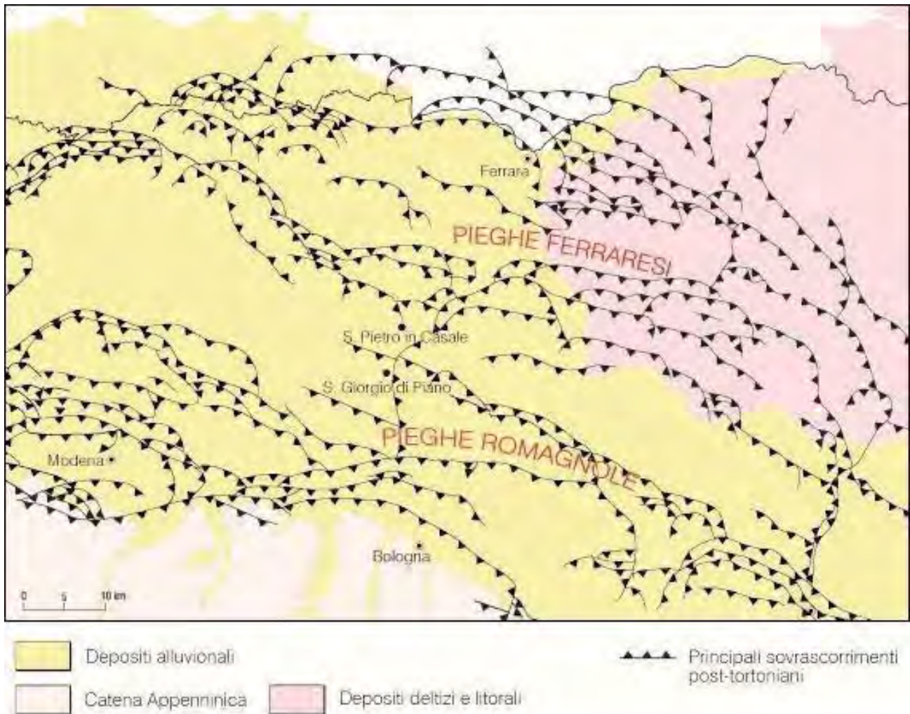
Figura 2-7 - Inquadramento tettonico illustrante la complessità delle strutture dell'arco delle Pieghe Romagnole e Ferraresi. Modificato dalle Note Illustrative del Foglio CARG 203, Poggio Renatico.
