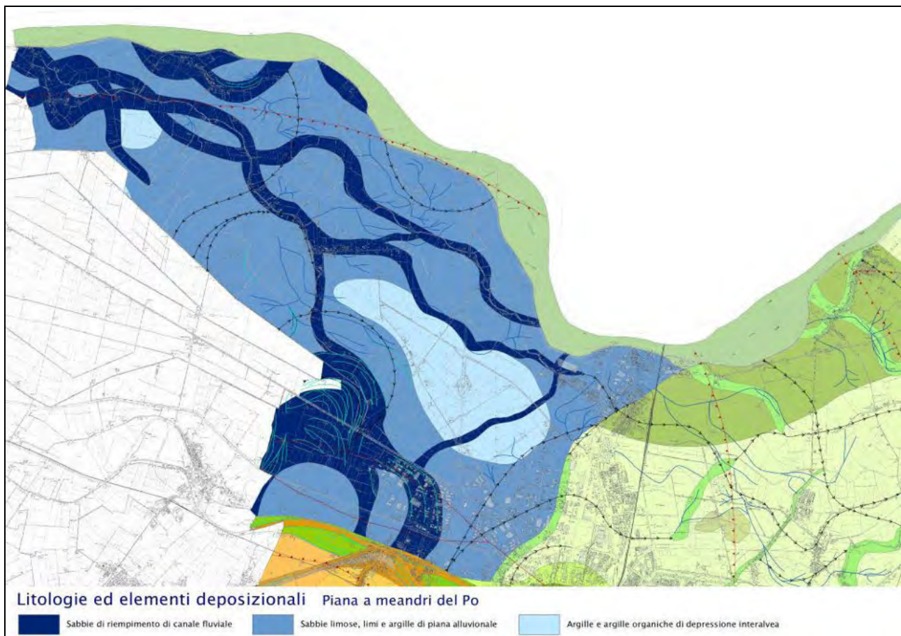
Figura 5-1 - Stralcio della carta geologica qui presentata, rappresentante la parte nord-occidentale del territorio comunale, dominata dalle sabbie di riempimento di canali a meandro del Po.
