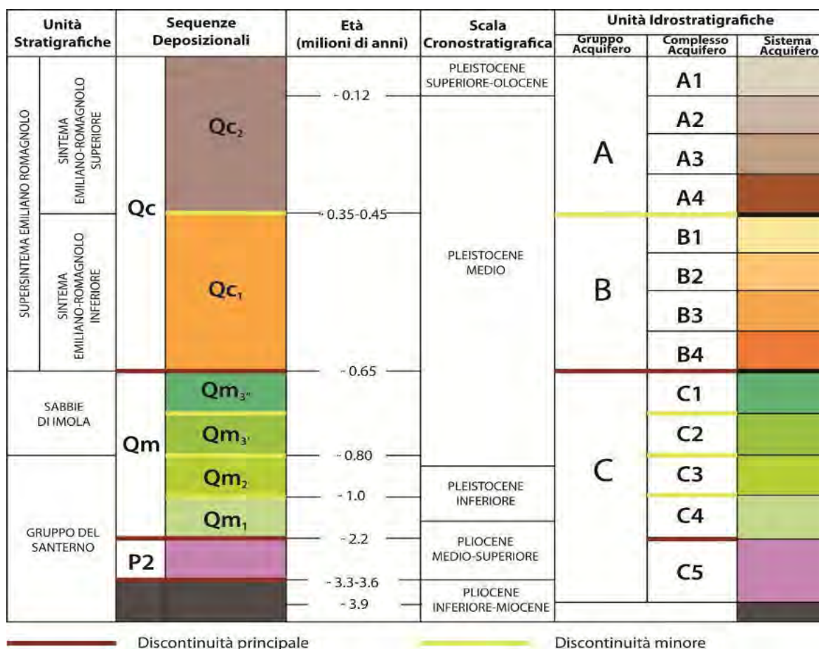
Figura 2-4 - Schema stratigrafico-sequenziale dei depositi plio-quaternari del bacino padano, con indicazione delle unità idrostratigrafiche. Regione Emilia-Romagna & Eni-Agip, 1998.
