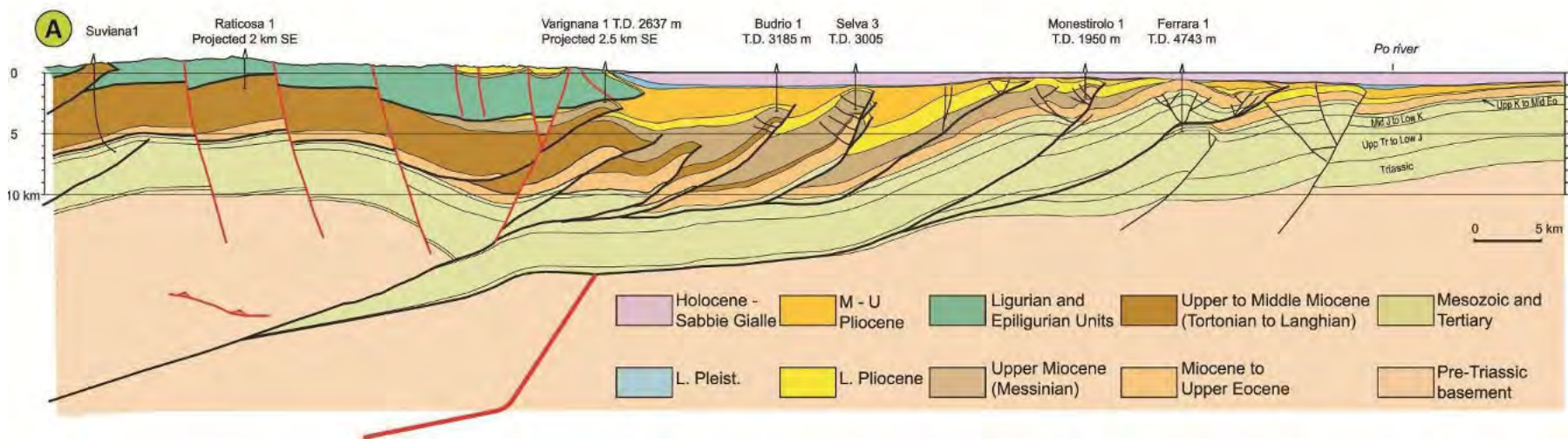
Figura 2-9 - Contesto strutturale della porzione emiliano-romagnola dell'Avanfossa Appenninica. La sezione superiore (B) da Pieri & Groppi, 1981 la sezione inferiore (A) da Toscani et al. , 2009.
