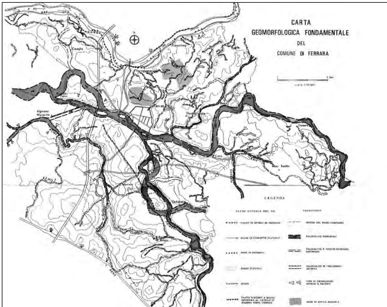
Figura 2-2 - Carta Geomorfologica Fondamentale derivate dallo "Studio geologico coordinato per la pianificazione territoriale del Comune di Ferrara" - Bartolomei et al. , 1975.
