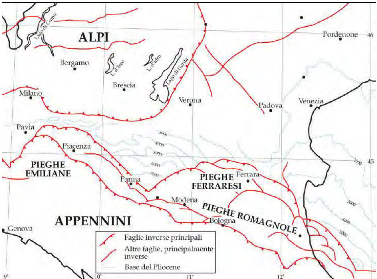
Figura 2-6 - Carta strutturale semplificata della Pianura Padana (Pieri & Groppi, 1975). Le isobate si riferiscono alla profondità della base dei sedimenti pliocenici. Modificata da Burrato et al. , 2003.
