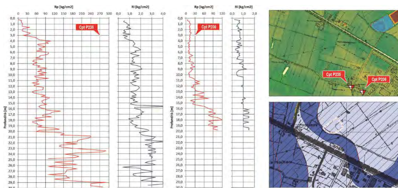
Figura 5-2 - Log parametrici di resistenza alla punta ( R_p ) e attrito laterale ( R_l ), relativi a due prove Cpt realizzate in prossimità del comparto 17ASPCN-01 del Piano Operativo Comunale di Ferrara. I grafici a sinistra descrivono la facies penetrometrica di corpi di riempimento di un meandro, quelli a destra i caratteri della piana interalvea adiacente.
