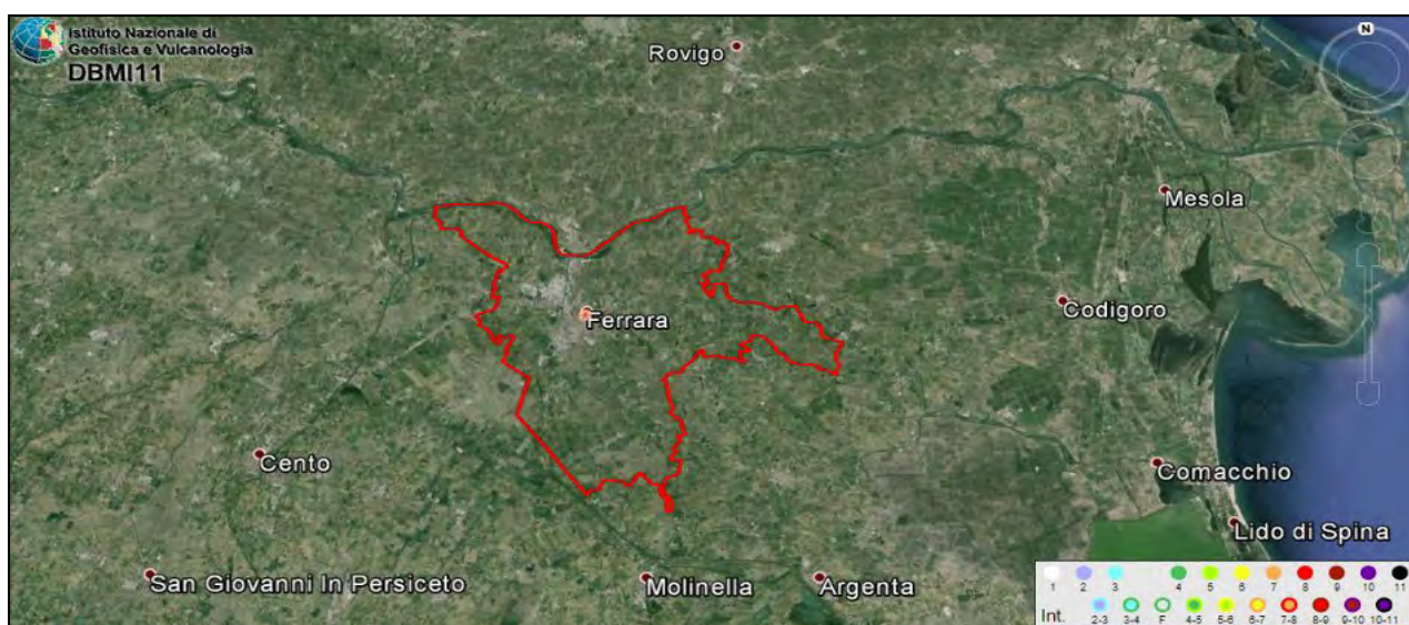
Figura 2-14 - Effetti del sisma del 9 gennaio 1411. Dati DBMI11. In rosso è rappresentata l'area del Comune di Ferrara.
