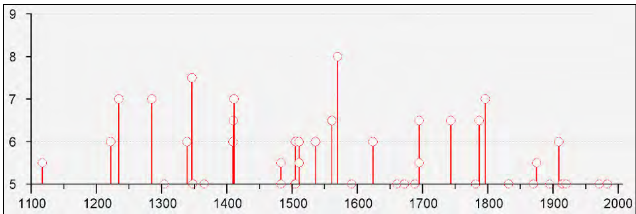
Figura 2-12 - Valori di intensità macrosismica I_{MCS} \geq 5 attribuiti al Comune di Ferrara, dall'anno 1000 al 2006, e legati essenzialmente ad eventi prodotti dalle strutture tettoniche ferraresi. Tratto dal database DBMI11 (Locati et al. , 2011).
