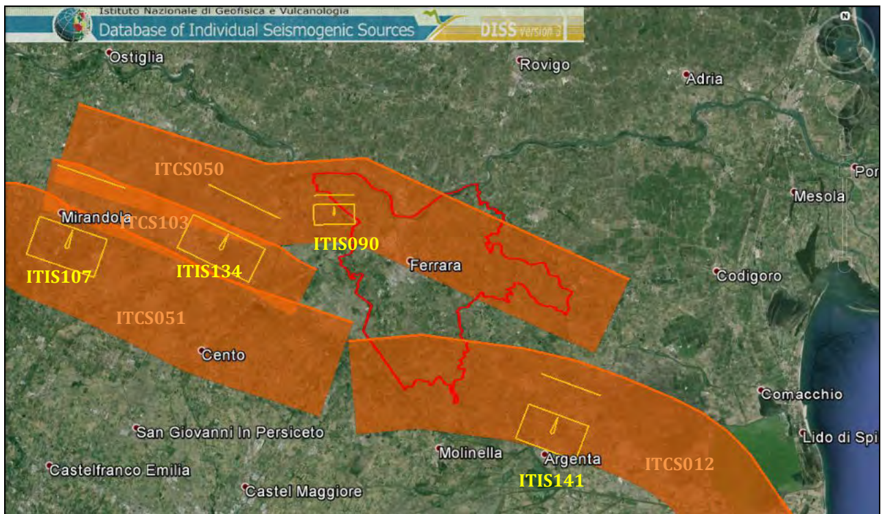
Figura 2-10 - Sorgenti sismogenetiche composite (poligoni arancioni) e individuali (rettangoli gialli) presenti nel database DISS 3.2.0, nell'intorno dell'area di studio. In rosso è riportata l'area occupata dal territorio del Comune di Ferrara.
