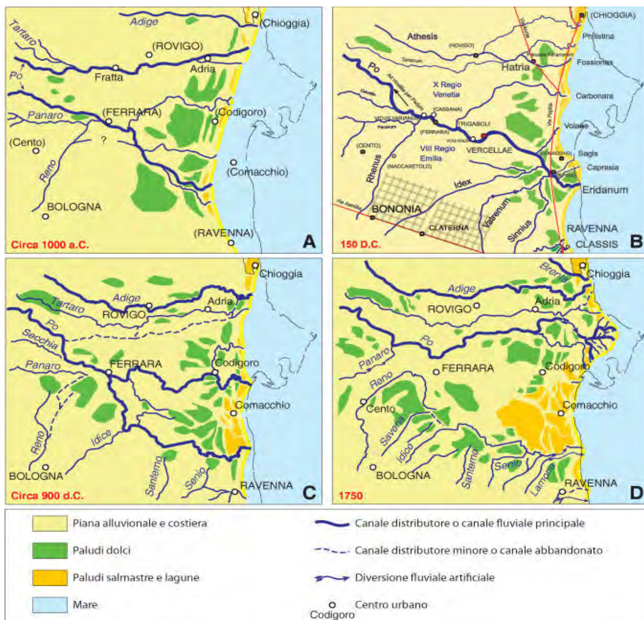
Figura 2-18 - Evoluzione del reticolo idrografico della fascia costiera negli ultimi 3000 anni. Da Bondesan, (1990) come modificate in Stefani & Vincenzi (2005).
