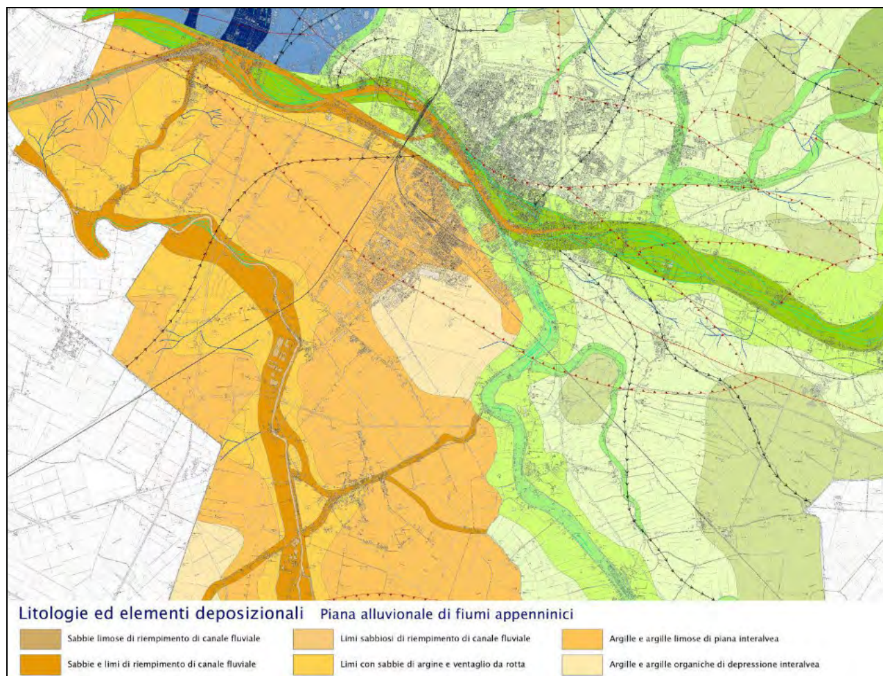
Figura 5-5 - Stralcio della carta geologica a sud del centro storico che illustra il grande corpo di paleoalveo del Fiume Reno, in gran parte deposto durante il XVII secolo. Notare l'accumulo di sedimenti di Reno entro l'precedente alveo del Po a sud e sud-ovest del centro storico.
