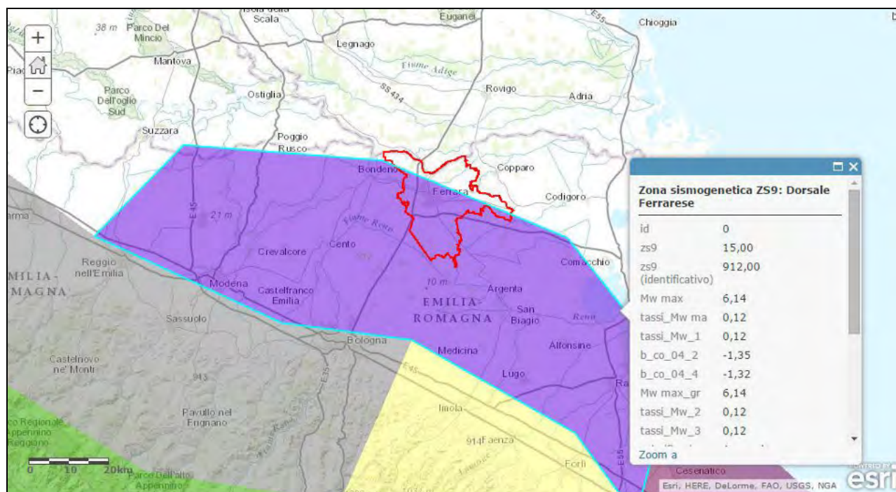
Figura 2-11 - Ubicazione del territorio del Comune di Ferrara (in rosso) rispetto alla zonazione sismogenetica ZS9 (Meletti e Valensise, 2004).
