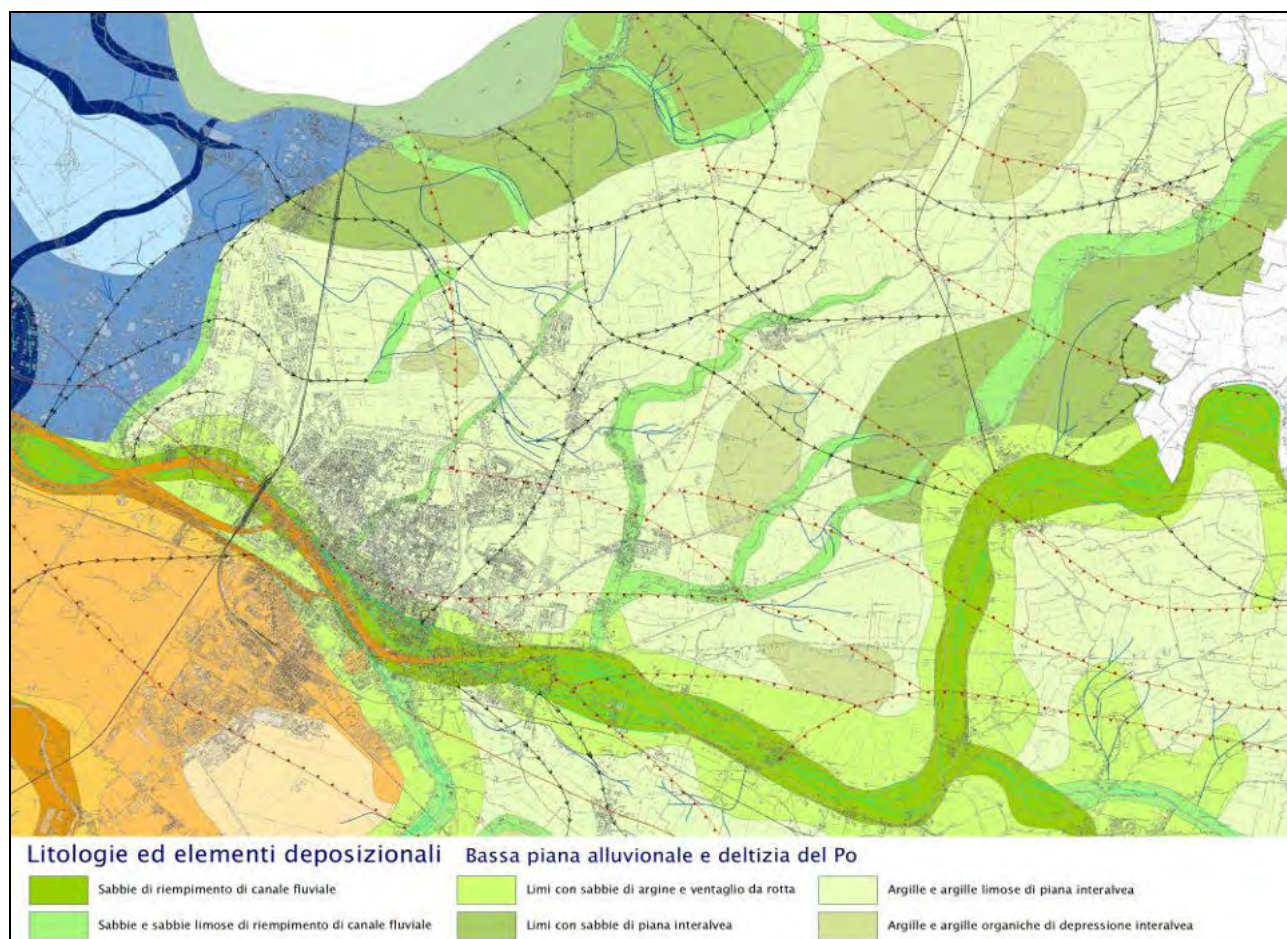
Figura 5-3 - Stralcio della carte geologica rappresentante il centro storico e la parte centro-orientale del territorio comunale, dominata da grandi corpi allungati di sabbie di canale di Po, fiancheggiati dai relativi corpi di argine naturale e da aree interalvee, ricchi di fanghi e torbe.
