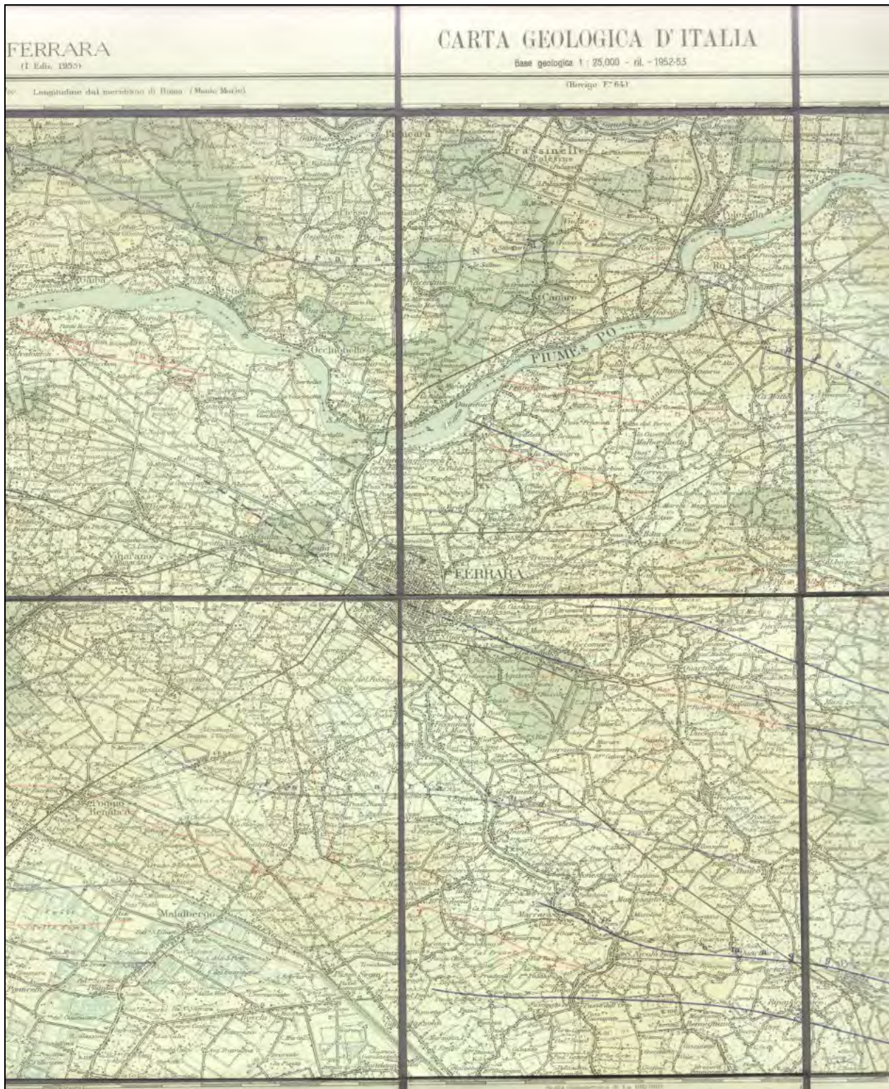
Figura 2-1 - Riproduzione della parte centrale del Foglio 76 "Ferrara" in scala 1:100.000 della Carta Geologica d'Italia, realizzata nel 1955 a cura del Servizio Geologico Nazionale.
