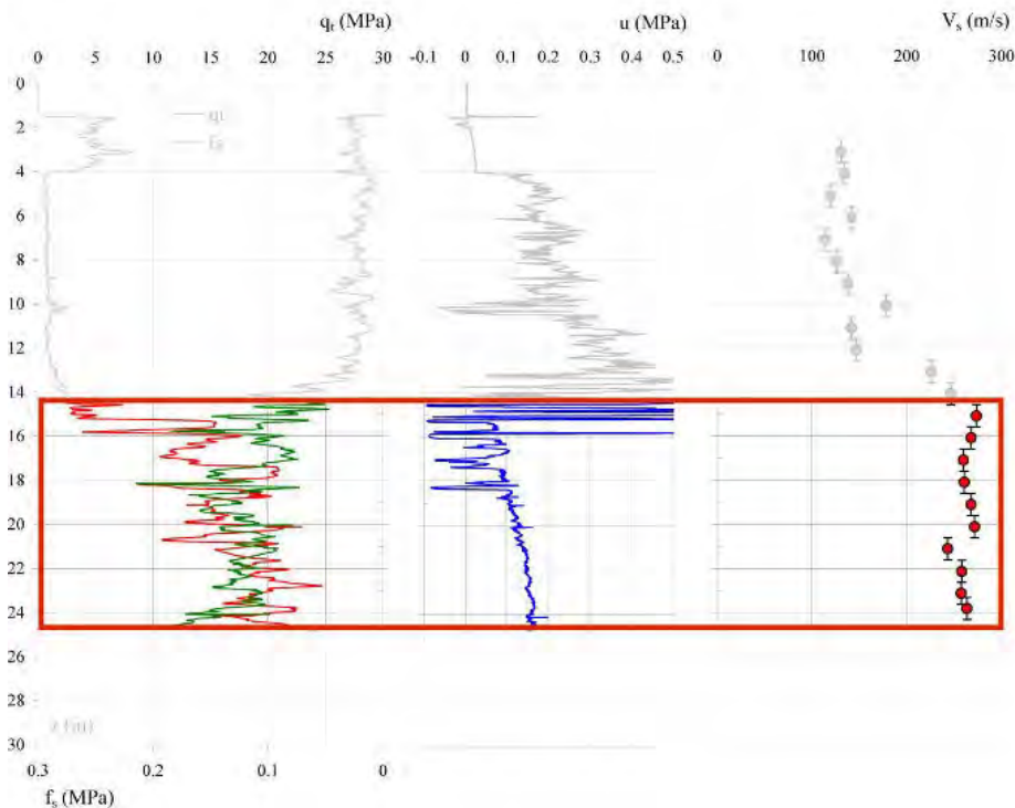
Figura 4-1 - Log parametrici di resistenza alla punta ( q_t ), attrito laterale ( f_s ), pressione neutra ( u ) e velocità delle onde sismiche seconde ( V_s ) relativi al piezocono sismico realizzato presso la scuola materna di Pontelagoscuro (FE). La porzione inferiore del grafico corrisponde alle sabbie singlaciali. Prova eseguita per la realizzazione del R.U.E. -Regolamento Urbanistico Edilizio di Ferrara.
