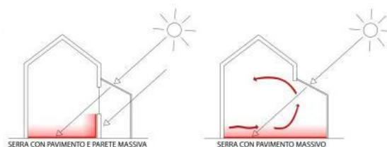
ESEMPI DI SISTEMI DI CAPTAZIONE SOLARE
