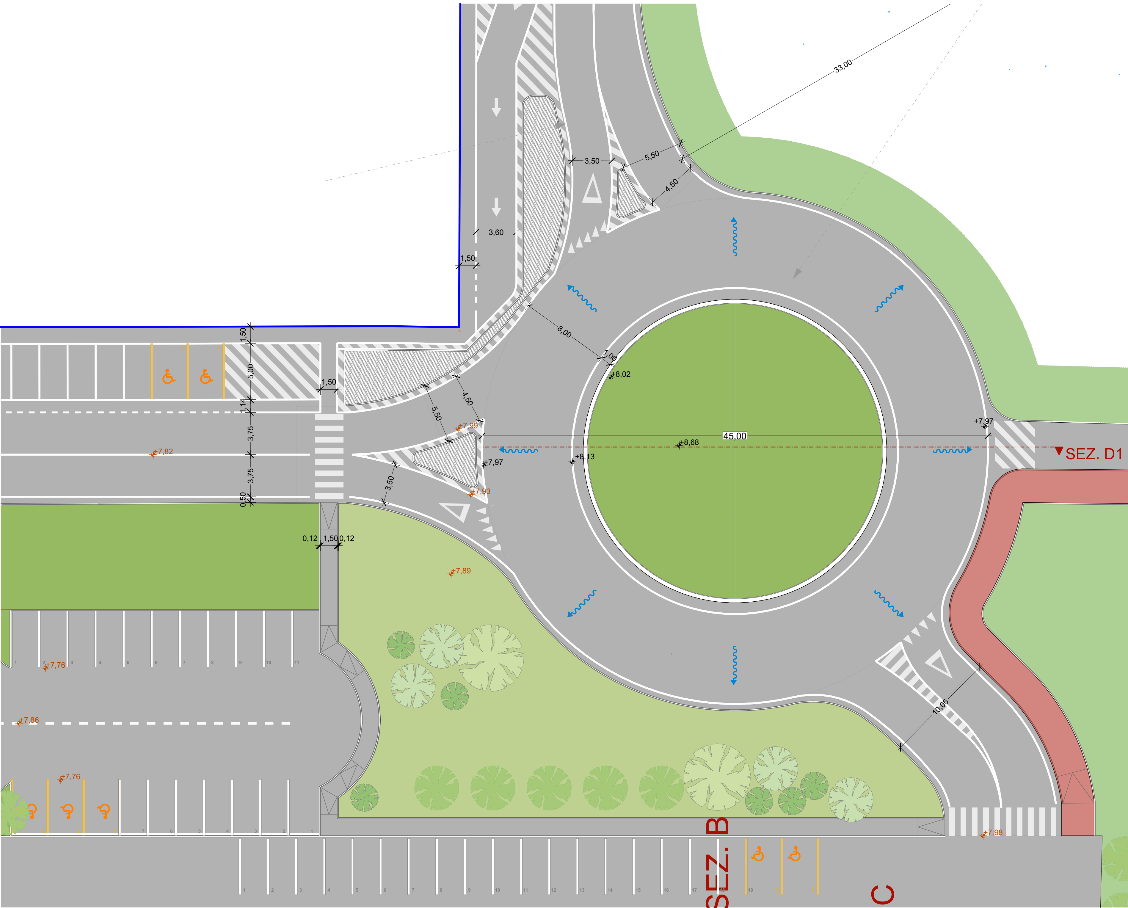
Planimetria area Rotatoria
