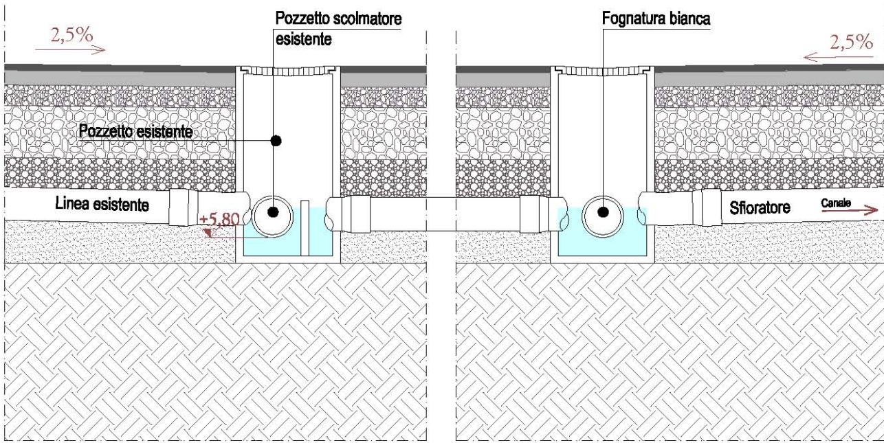
Dettaglio pozzetti di raccordo. Scala 1:25
